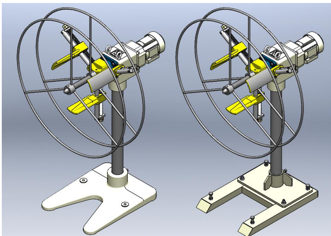
鋳造製 (変更前)
