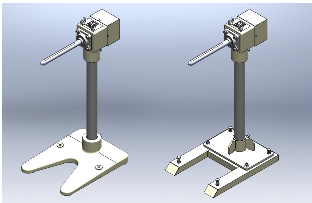
鋳造製（変更前）
